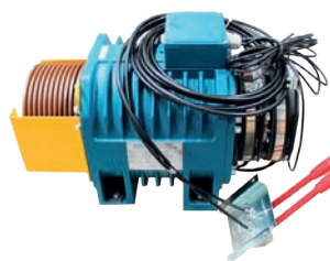
Máquina de tracción gearless 1000 kg, 1.6 m/s, 10.2 Kw
