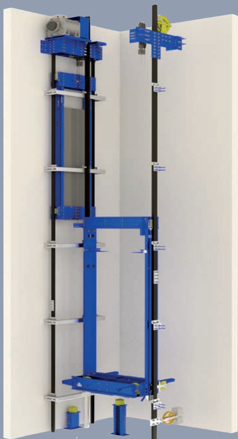
MRL-G: Modelo de chasis de cabina G.
