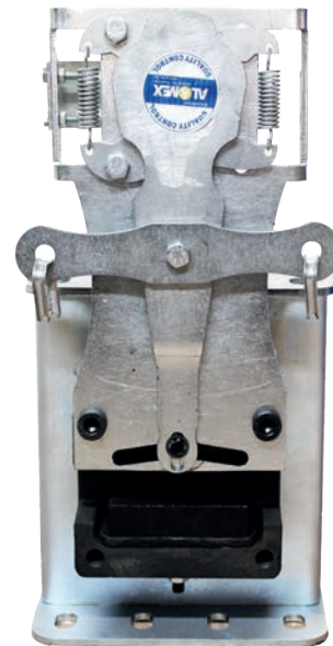
Paracaídas progresivo 2500 Kg ajustable 9 mm a 16 mm
