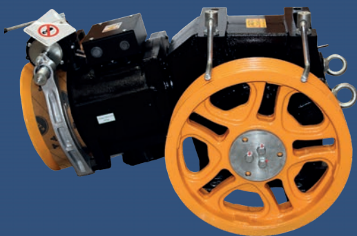
Máquina de tracción con engrane 1000 kg, 1.6 m/s, 13.5 Kw
